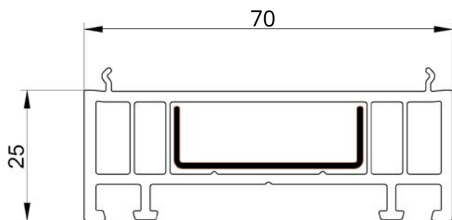
PVC PROFIL PROŠIRENJE BW 5031
