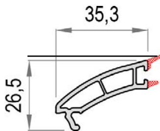
PVC LAJSNA BW 7053
