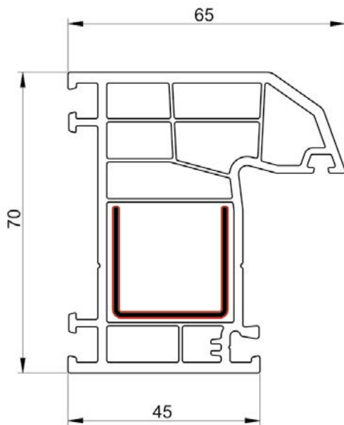
PVC PROFIL ŠTOKA BW 7001
