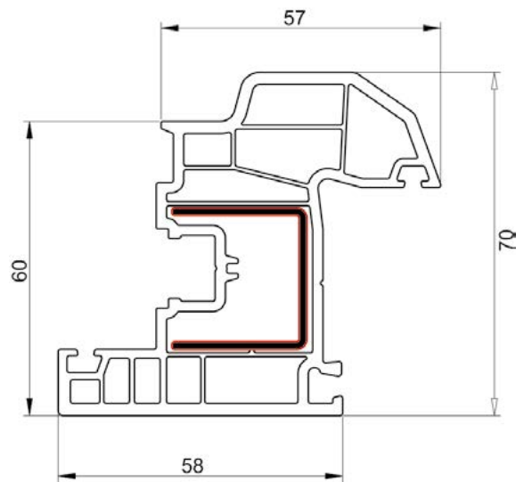
PVC PROFIL KRILO PROZORA BW 7011
