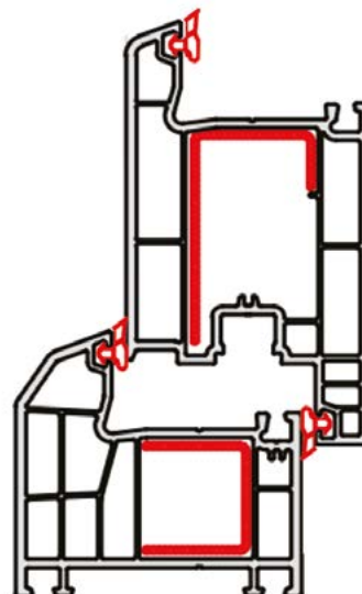
SISTEM VRATA
