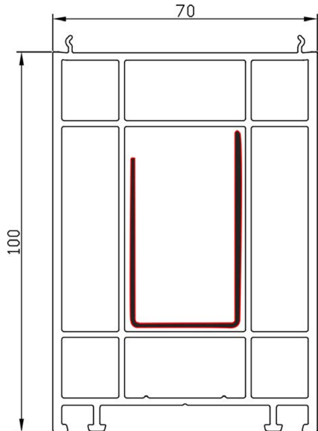
PVC PROFIL PROŠIRENJE BW -
